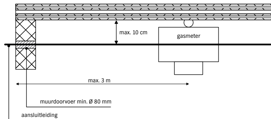
Juiste positie van de muurdoorvoer
